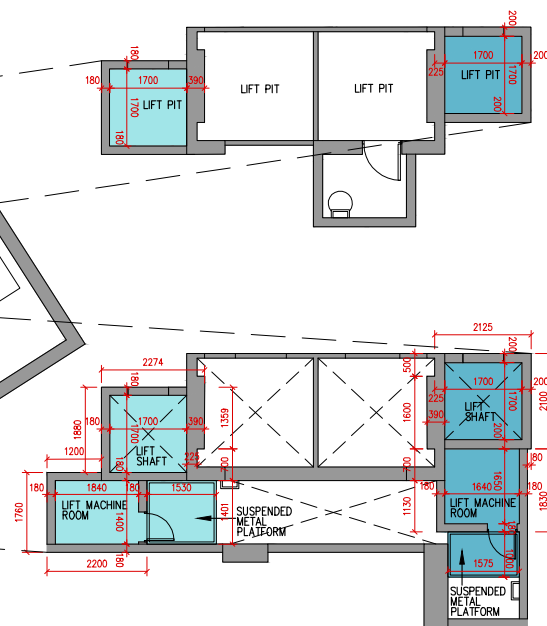
地庫升降機槽底部份平面圖
