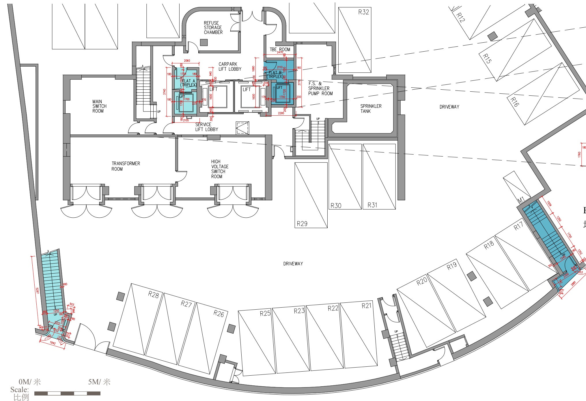
地庫層平面圖
